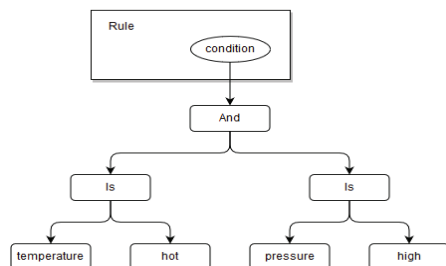
Рис. 1. Пример древовидной структуры правила (Rule)
