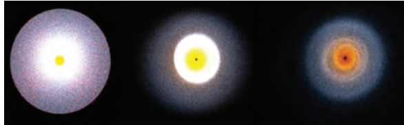
Рисунок 4 – Динамика экспоненциального диска в самосогласованном поле.
