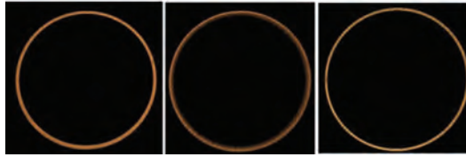
Рисунок 3 – динамика кольца плотности в поле массивного тела.
