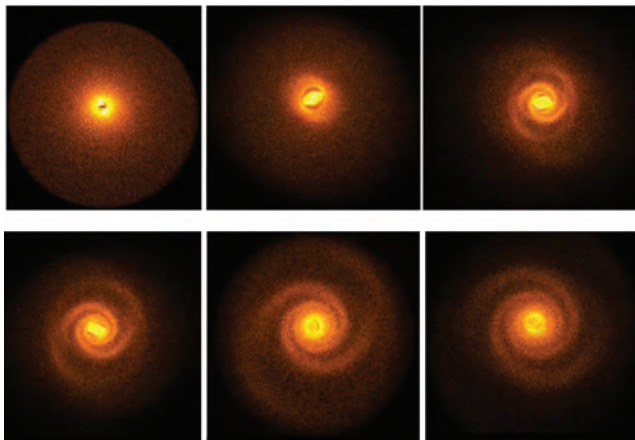
Рисунок 5 – эволюция экспоненциального диска в различных моменты времени.
