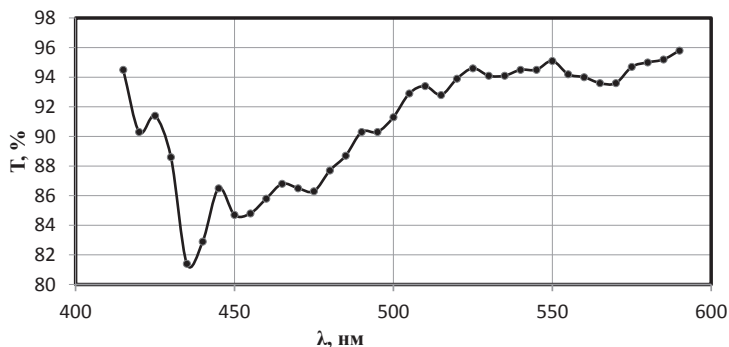
Рисунок 1 – Характеристика, фиксируемая на спектрофотометре.
