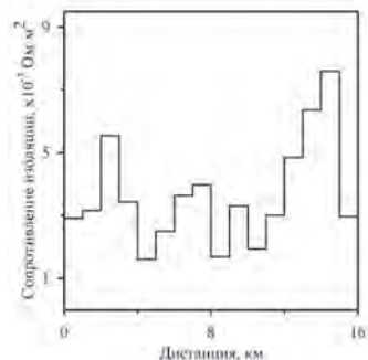
Рис. 2. Расчет: сопротивление изоляции на защищаемом участке трубопровода.
