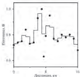
Рис. 1. Аппроксимация потенциала вдоль трубопровода; точки – данные измерений.
