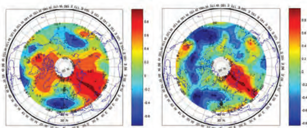
Рисунок 1 – Пространственное распределение корреляционных связей по северному полушарию. Реперная точка \lambda = 50^\circ в. д.
