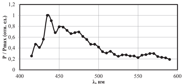
Рисунок 2 – Излучательная способность лазера.
