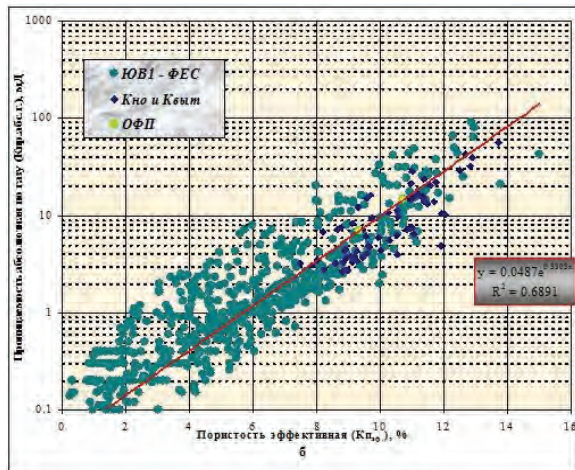
Рис. 1 (б). – Результаты сопоставления данных по абсолютной проницаемости и эффективной пористости (б) с информацией по охарактеризованности специальными петрофизическими исследованиями ( K_{но} и K_{выт} , ОФП, капилляриметрии) относительно всего массива данных пласта ЮВ 1 Лас - Еганского месторождения
