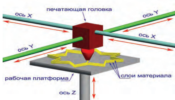
Рис. 2 Схематическое изображение 3D – принтера
