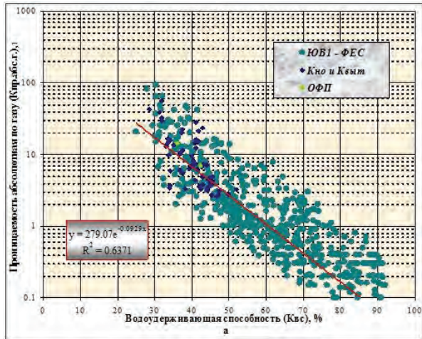
Рис. 1 (а). – Результаты сопоставления данных по абсолютной проницаемости с водоудерживающей способностью с информацией по охарактеризованности специальными петрофизическими исследованиями ( K_{но} и K_{выт} , ОФП, капилляриметрии) относительно всего массива данных пласта ЮВ 1 Лас - Еганского месторождения
