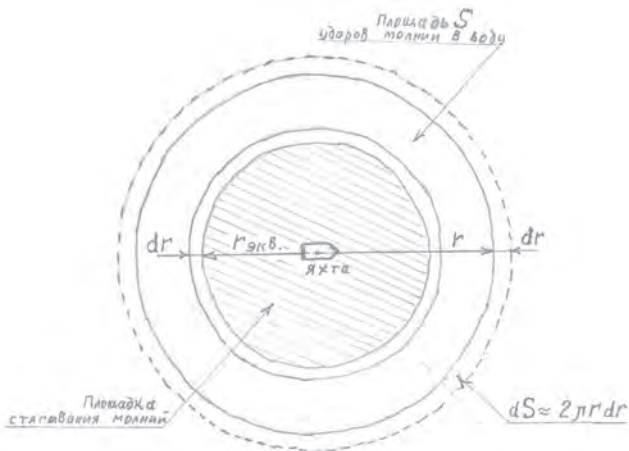
Рисунок 1. К расчету числа опасных близких ударов молнии в воду.
