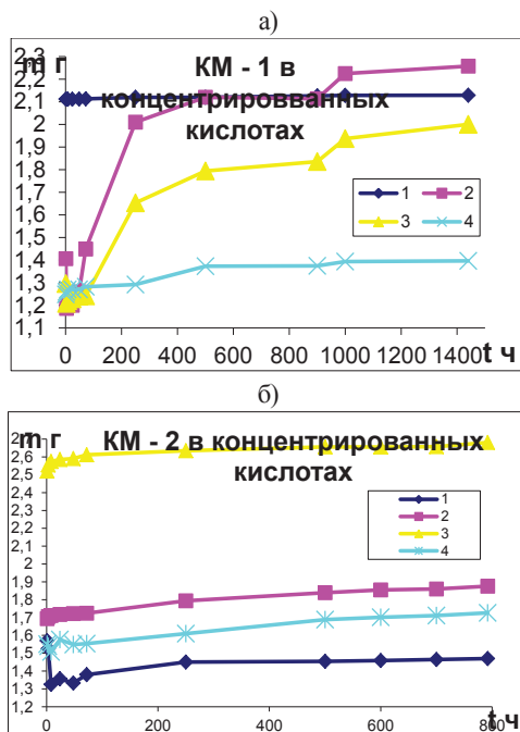
Рис.1а, б. Изменение массы опытных образцов в концентрированных кислотах в зависимости от времени выдержки:
