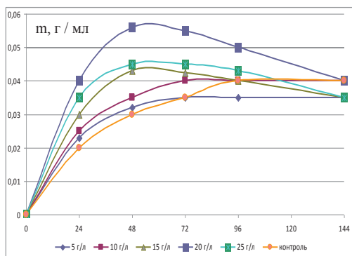
Рис. 1. Исследование процессов роста лактобактерий на среде с изомальтулозой в различной концентрации
