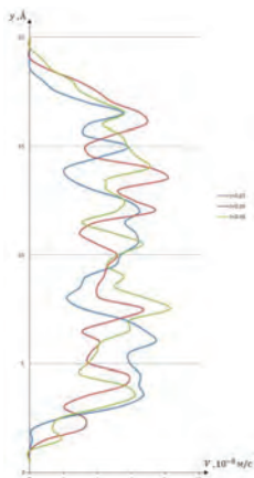
Рис.2 Распределение средней скорости молекул в сечении канала.
