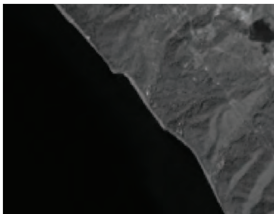
Рисунок 1 – Фрагмент снимка Landsat 8 (составлен автором)
