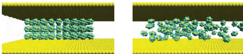
Рис.1 Эволюция облака молекул циклогексана
