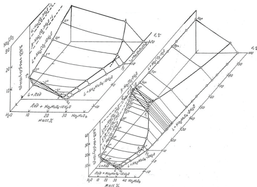
Рисунок. Изобарно - политермическая диаграмма растворимости в системе карбонат натрия - молибдат натрия - вода.
