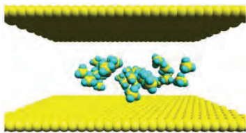
Рис.2. Движение молекул метана в сдвиговом потоке.
