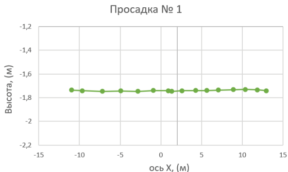
Рисунок 3 – Диаграмма просадки № 1 плит перекрытий здания
