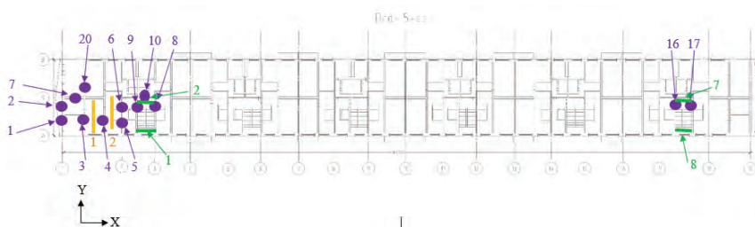
Рисунок 2. План - схема 5 этажа здания с указанием мест проведения геодезических измерений
