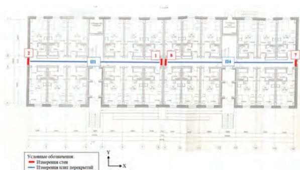
Рисунок 1 – Схема проведения геодезической съёмки здания
