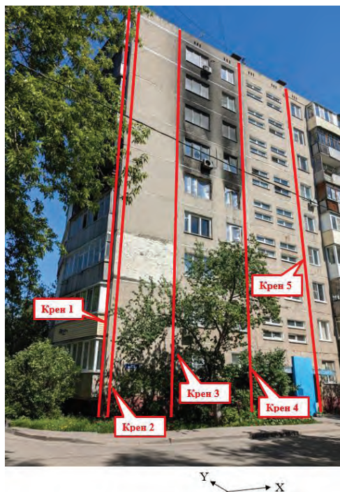
Рисунок 1 – Схема проведения геодезической съёмки здания (красным показаны крены здания)
