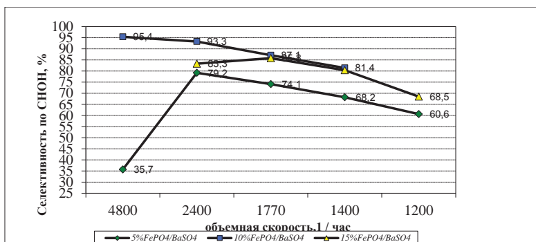
Рис.2. Зависимость селективности по формальдегиду от скорости пропускания метана ( T=943\text{K} , [\text{CH}_4]:[\text{O}_2] = 1:1 ).
