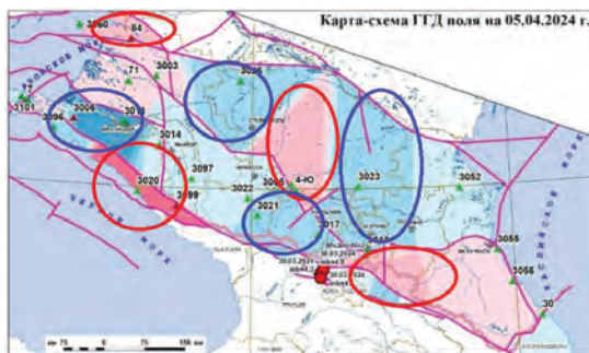
Рисунок 1 – Схема расположения зон сжатия и растяжения земной коры на территории Кавказа (по данным «Гидроспецгеологии») (красным - зона сжатия, синим - зона растяжения)
