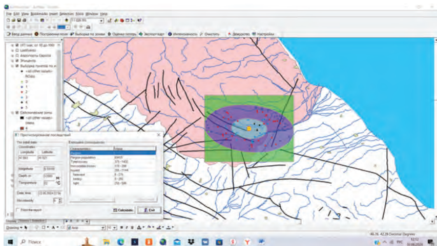
Рисунок 1 – Моделирование сценарного землетрясения на территории Кавказа
