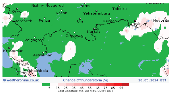
Рисунок 5. Карта вероятности грозы от 20.05.2024. Грозовая активность присутствует на территории Кавказа.
