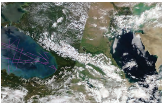
Рисунок 4. Портрет облачности на Кавказе и его окрестностях (Спутниковый снимок «Suomi NPP» от 03.04.2024)
