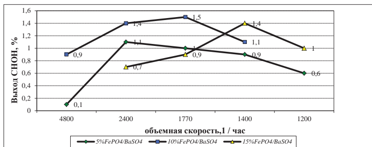
Рис.1. Зависимость выхода формальдегида от объемной скорости по метану ( T=943\text{K} , [\text{CH}_4]:[\text{O}_2] = 1:1 ).
