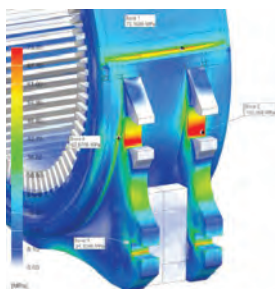
Рис. 4 – Напряжения в кронштейне колебательного подвеса тягового электродвигателя
