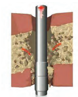
Рисунок 2 – обрушение стены скважины
