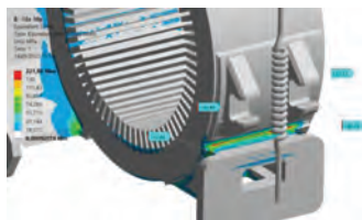
Рис. 2 – Напряжения при нагрузке в кронштейне колебательного подвеса электрического двигателя
