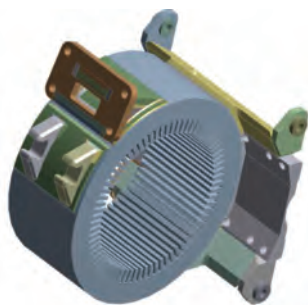
Рис. 1 – Пространственная детальная модель тягового электрического двигателя
