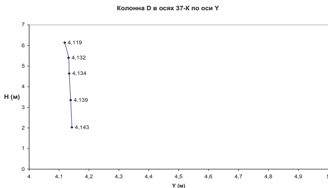
Рисунок 4. Диаграмма отклонения колонны № 4
