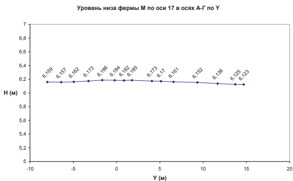
Рисунок 1. Диаграмма отклонения фермы № 1
