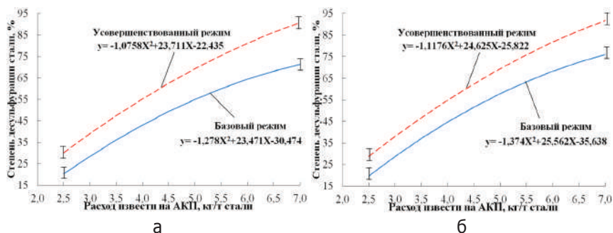
Рисунок 2. Степень десульфурации сталей Ш2.1 (а) и Ш2.3 (б) в зависимости от режима обработки на агрегате «ковш - печь»
