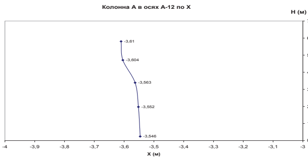
Рисунок 1. Диаграмма отклонения колонны № 1
