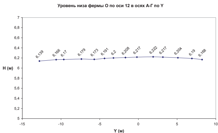
Рисунок 3. Диаграмма отклонения фермы № 3
