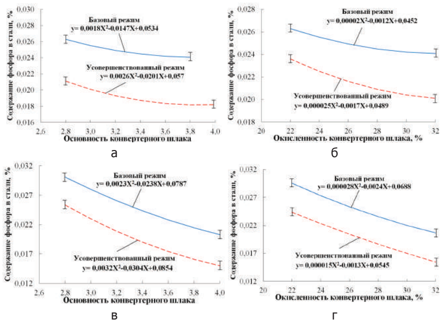
Рисунок 1. Влияние режимов конвертерной плавки на содержание фосфора в стали в конце продувки
