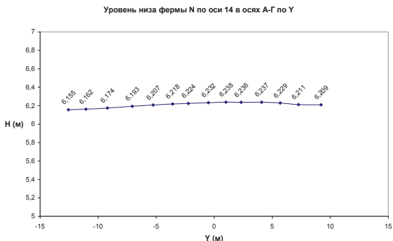
Рисунок 2. Диаграмма отклонения фермы № 2
