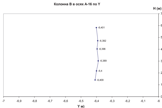
Рисунок 3. Диаграмма отклонения колонны № 3
