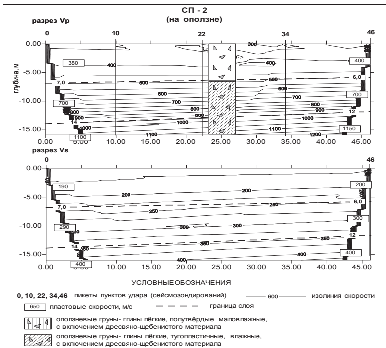
Рисунок 4 – Разрезы скоростей сейсмических волн КМПВ
