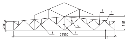
Рисунок 1 – Стальные фермы
