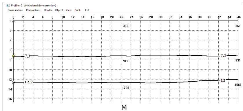
Рисунок 3 – Геосейсмический разрез КМПВ
