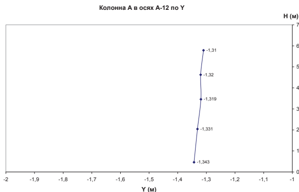
Рисунок 2. Диаграмма отклонения колонны № 2
