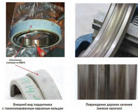
Рисунок 1 – Бринеллирование шарикового подшипника с приводной стороны электродвигателя
