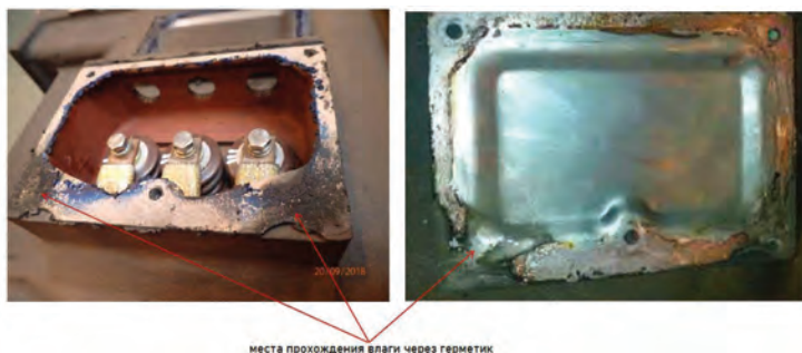
Рисунок 2 – Конструктив крышки клеммной коробки
