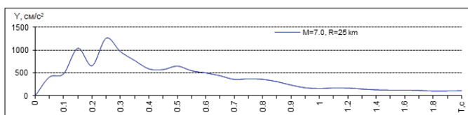
Рисунок 5 – Расчётный спектр реакции
