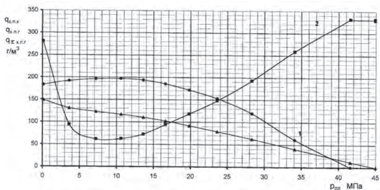
1 – пластовые потери конденсата ( q_{к.п.л.} ), 2 – содержание конденсата в пластовом газе ( q_{к.п.г.} ); 3 – суммарная добыча конденсата ( q_{к.п.г.} )
