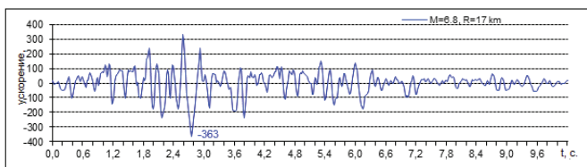
Рисунок 4 – Расчётная акселерограмма с дневной поверхности
