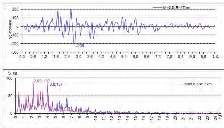
Рисунок 2 – Исходные акселерограммы и их спектры
