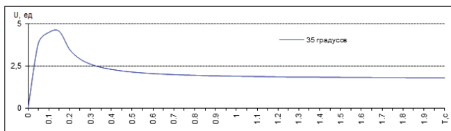
Рисунок 3 – Расчётная спектральная характеристика грунтового массива
