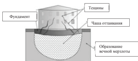
Рисунок 1 – Образование чаши оттаивания под зданием
