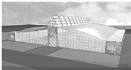
Рис. 2. Двухпролетное линзообразное мембранно - пневматическое сооружение
