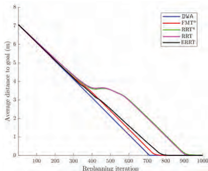
Рис.3. Текущее расстояние до цели по сравнению с итерацией повторного планирования.
