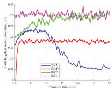
Рис.2. Отклонение от начального маршрута
