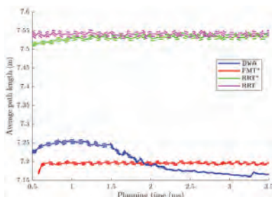
Рис.2. Средняя длина пути и максимально допустимое время планирования. Пунктирная линии представляют верхний и нижний крайние значения 95 % доверительного интервала.
