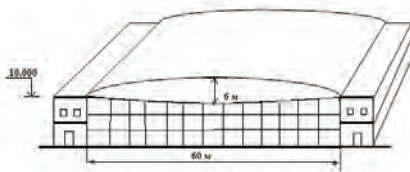
Рис. 1. Мембранно - пневматическое здание пролетом 60 метров
