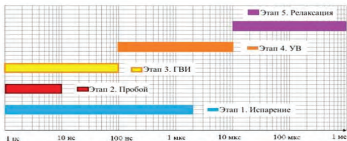
Рисунок 1 - Длительность этапов развития импульсного оптического разряда
