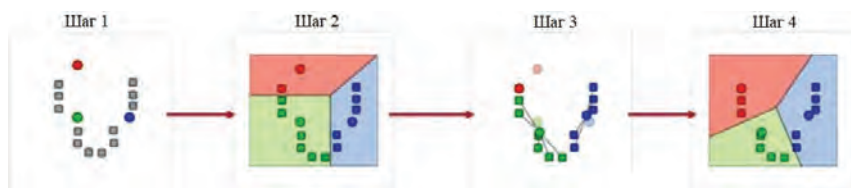
Рисунок 1. Схема реализации метода К средних (K-means)
