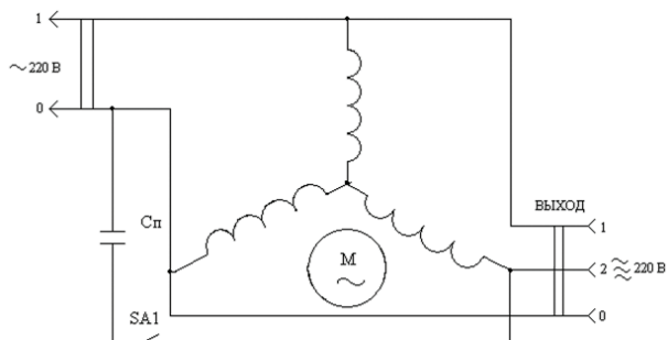
Рисунок 1. Схема преобразователя на "трёхфазное" линейное напряжение 220 В
