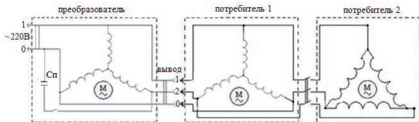
Рисунок 3. Подключение потребителей к преобразователю
