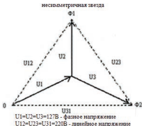
Рисунок 2. Векторные диаграммы напряжений вырабатываемые преобразователем
