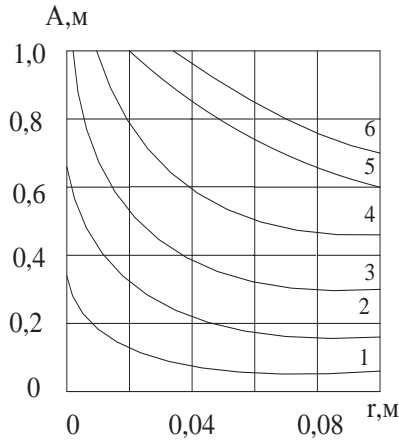
Рисунок 2. Влияние радиуса канала на величину термического сопротивления пода при высоте каналов 0,25r и шаге их расположения 0,2m : 1 - \delta = 0,05; 2 - 0,15; 3 - 0,25; 4 - 0,35; 5 - 0,45; 6 - 0,50m
