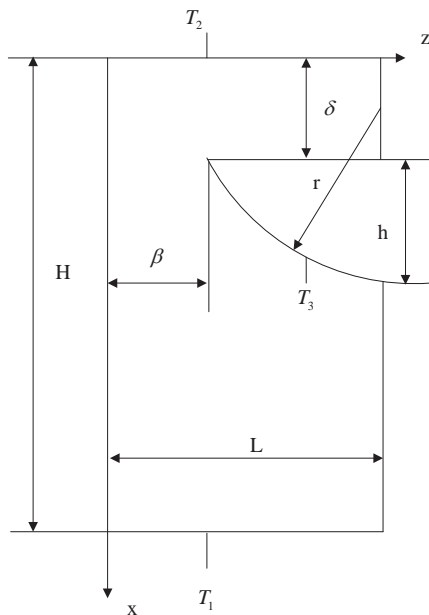
Рисунок 1. Расчетная схема
