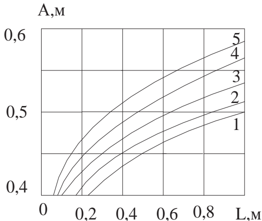
Рисунок 3. Влияние радиуса канала на величину термического сопротивления пода при глубине заложения каналов 0,25m и их радиусе 0,08m : 1 - h = 0,25; 2 - 0,5; 3 - 1,0; 4 - 1,5; 5 - 2r ; (круглый канал).
