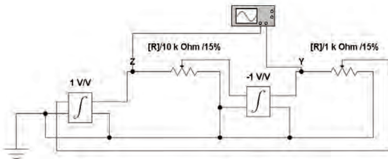
Рисунок 1. Схема набора модели для воспроизведения функций y = A\sin(\omega t + j) и z = A\cos(\omega t + j)
