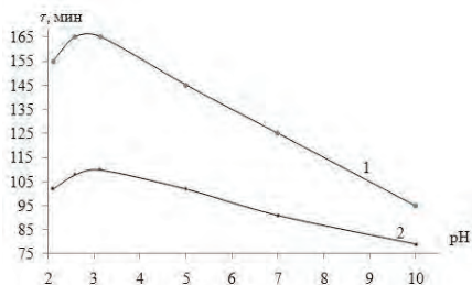
Рис. 1. Зависимость между временем устойчивости TCNE: 1 - водного раствора, 2 - в диоксане и кислотностью раствора
