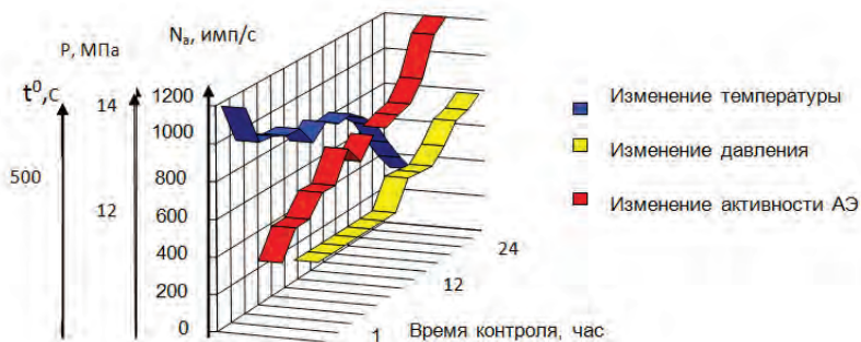
Рисунок 1 – Изменение технологических параметров паропровода и сигналов АЭ
