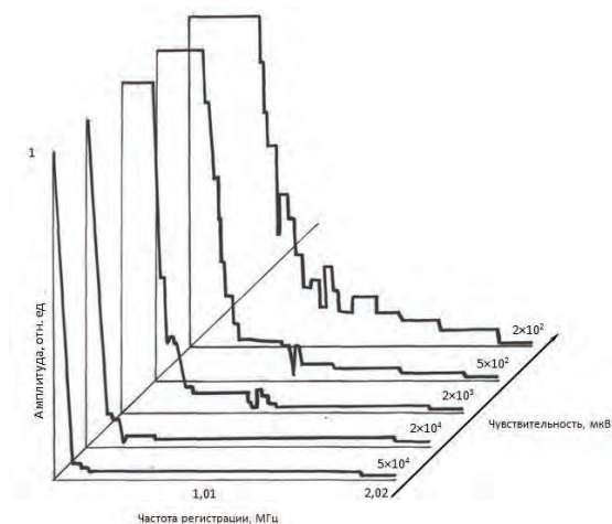
Рисунок 3 – Амплитудно - частотное распределение сигналов АЭ при регистрации технологических шумов в зависимости от чувствительности анализатора спектра
