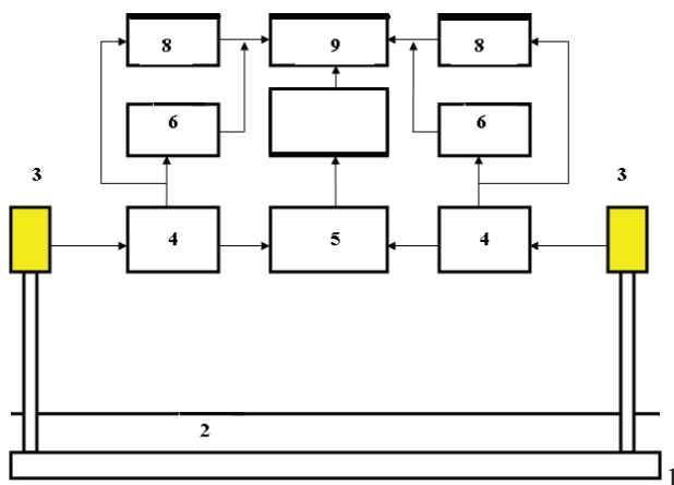
Рисунок 5 - Блок - схема регистратора сигналов АЭ с линейной локацией 1 – паропровод, 2 – изоляционный слой, 3 – преобразователи и предварительные усилители, 4 – основные усилители, 5 – блок обработки сигналов, 6 – сумматоры, 7 – блок определения координат, 8 – интенсиметры, 9 – цифровое табло и определитель координат
