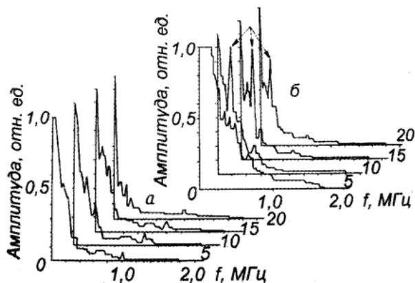
Рисунок 4 – Амплитудно - частотное распределение сигналов АЭ на бездефектном (а) и участке с повышенной активностью (б), указано стрелками
