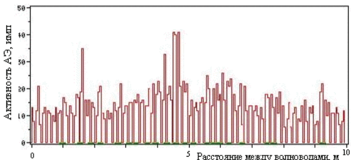
Рисунок 6 - Активность сигналов АЭ при линейной локации
