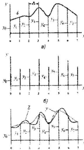
Рисунок 1 - Интерполяция:
