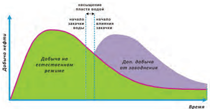
Рисунок 1. График влияния дополнительной закачки воды на добычу
