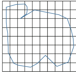
Рисунок 2. матрица пласта
