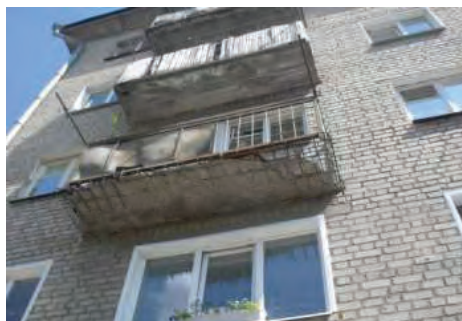
Рисунок. Разрушение консольной балконной плиты жилого здания
