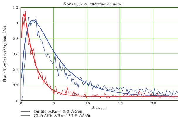
Рисунок 1. Выделение радона из золы - унос и цемента в водопроводную воду
