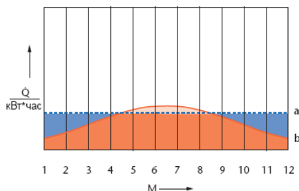
Рисунок 1. Соотношение между выработкой энергии гелиоколлекторной установкой и годовой потребностью в тепловой энергии для ГВС.
