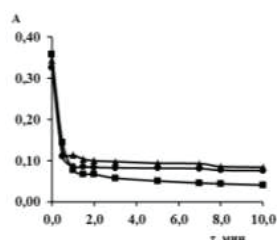
Рис. 2. Изотермы кинетики сорбции ионов цинка сорбентом СВ - 1 - К: - \Delta - 277 К; - \square - 298 К; - \circ - 313 К
