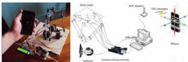
Рисунок 4 - Дельта - робот, управляемый с помощью акселерометра iPhone
