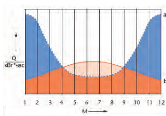
Рисунок 2. Соотношение между выработкой энергии гелиоколлекторной установкой и годовой потребностью в тепловой энергии для ГВС и отопления.
