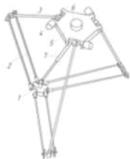
Рисунок 2 - Структурная схема механизма типа DELTA
