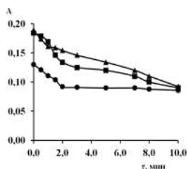
Рис. 1. Изотермы кинетики сорбции ионов цинка сорбентом СВ - 1 - А: - \Delta - 277 К; - \square - 298 К; - \circ - 313 К
