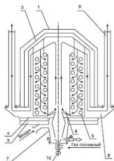
Рисунок 2. Схема теплообменной камеры печи ПТБ - 10А
