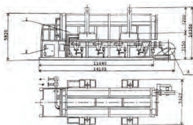
Рисунок 1. Составные блоки трубчатой печи ПТБ - 10А
