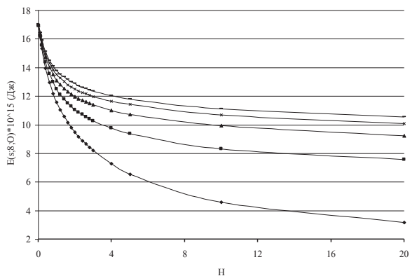
Рис. 6. Энергии, уносимые атомами из систем. r = 8 .
