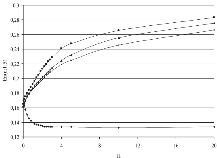
Рис. 7. Нормированные средние энергии, уносимые атомами из систем в зависимости от количества столкновений со стенками систем. r = 1 . \theta = 5^\circ .
