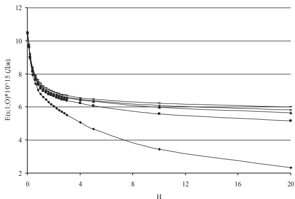
Рис. 5. Энергии, уносимые атомами из систем. r = 1 .
