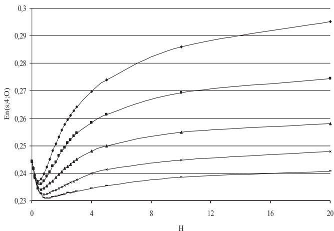
Рис. 3. Нормированные средние энергии атомов, вылетевших из систем. r = 1 . \blacklozenge – 0^\circ , \blacksquare – 5^\circ , \blacktriangle – 10^\circ , \times – 15^\circ , \cdot – 20^\circ .
