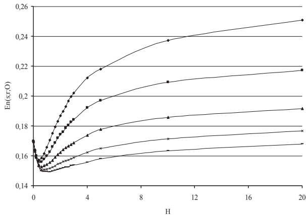
Рис. 2. Нормированные средние энергии атомов, вылетевших из систем. r = 1 . ◆ — 0^\circ , ■ — 5^\circ , ▲ — 10^\circ , × — 15^\circ , — — 20^\circ .
