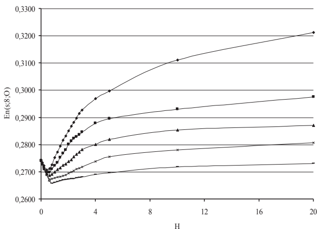
Рис. 4. Нормированные средние энергии атомов, вылетевших из систем. r = 8 . \blacklozenge – 0^\circ , \blacksquare – 5^\circ , \blacktriangle – 10^\circ , \times – 15^\circ , \cdot – 20^\circ .
