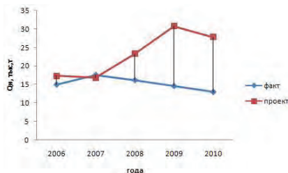
Рис.2 Показатели Q_n пласта Т на Западно - Кораблевском поднятии
