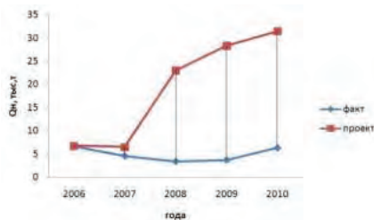
Рис.1 Показатели Q_n пласта Т на Кудрявцевском поднятии
