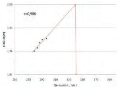
Рис.3 График зависимости логарифма обводненности от накопленной добычи нефти пласта Т на Кудрявцевском поднятии
