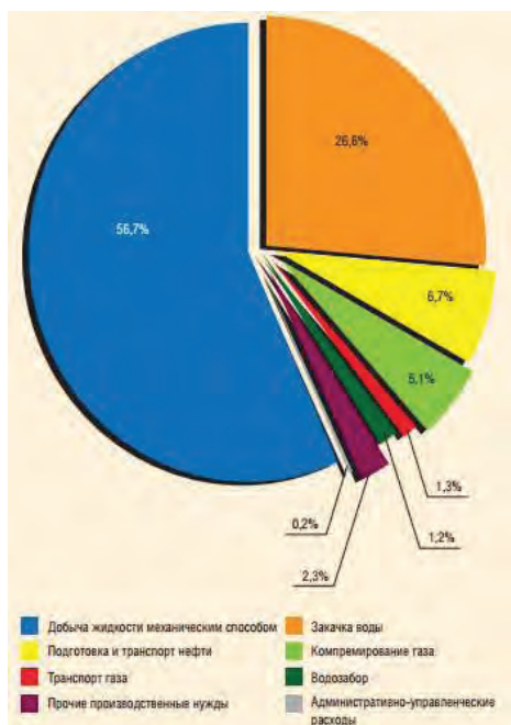
Рисунок 1. Распределение потребления энергии по технологическим процессам
