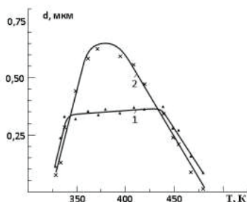
Рис.2. Зависимость толщины пленок теллура от температуры подложки:
