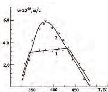
Рис.1. Зависимость скорости роста пленок теллура от температуры подложки:
