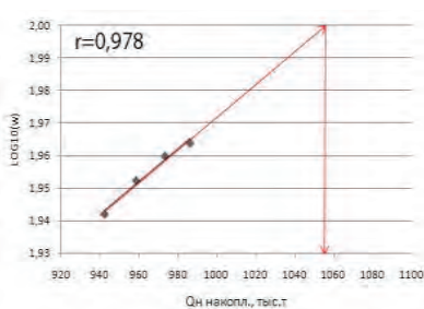
Рис.4. График зависимости логарифма обводненности от накопленной добычи нефти пласта Т на Западно - Кораблевском поднятии
